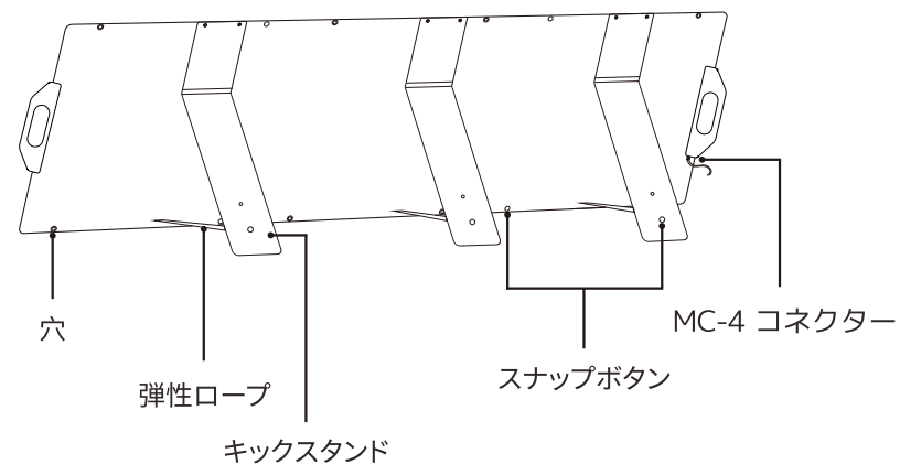
ソーラーハネル背面:
